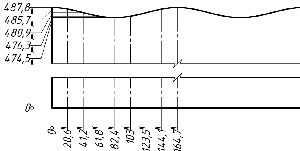
Поз.4 (Стойка) Развертка 1 : 3
